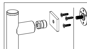
639 RZP ΡΟΖΕΤΑ ΛΑΒΗΣ ΕΞΩΠΟΡΤΑΣ PULL HANDLES ROSETTE
